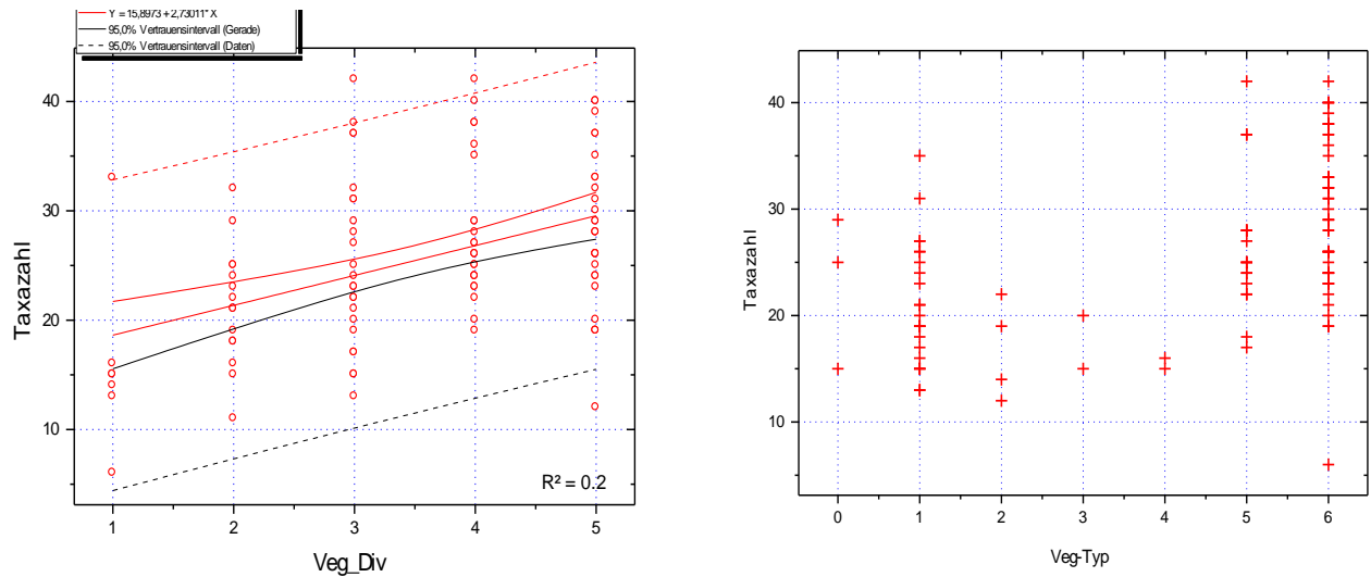
Abb. 25: Darstellung Zusammenhang zwischen Vielfalt und „Typ“ der submersen Vegetation (Veg.-Div., Verg.-Typ) und Makrozoobenthos-Taxazahl. Datengrundlage: Wesermarschuntersuchungen, Claus et al. (1994). Veg.-Div: 1 = niedrig – 5 sehr hoch. Veg.-Typ. 0 = keine Vegetation, 1 = Wasselinsen dominiert, 2= Fadenalgen, 3 = Röhricht, 4 = Enteromorpha, 5 = Wasserpest dominiert, 6 = verschiedene Arten (Laichkräuter, Hornkraut etc..)
