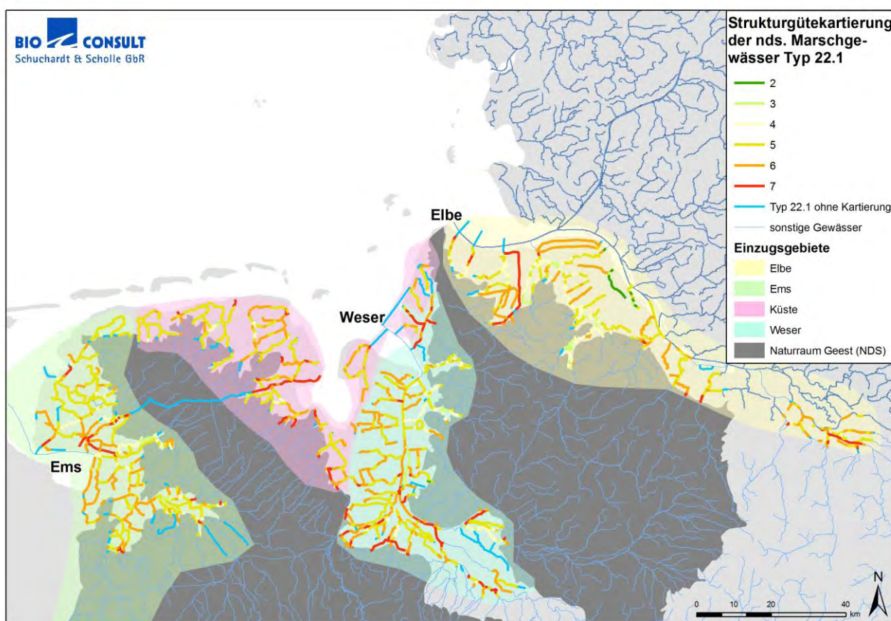
Abb. 5: Ergebnisse der Strukturgütekartierungen in den niedersächsischen Marschengewässern (Typ 22.1, nicht tideoffen). Daten NLWKN Stade. Bezeichnung: 7 = vollständig verändert, 6 = sehr stark verändert, 5 = stark verändert, 4 = mäßig verändert, 3 = deutlich verändert, 2 = gering verändert. Schwarze Punkte Makrozoobenthos-Messstellen. Graue Bereiche und Bereiche mit abgedunkelter Farbgebung spiegeln den Naturraum Geest wider. Abgrenzung des Naturraums Geest nur für Niedersachsen.
