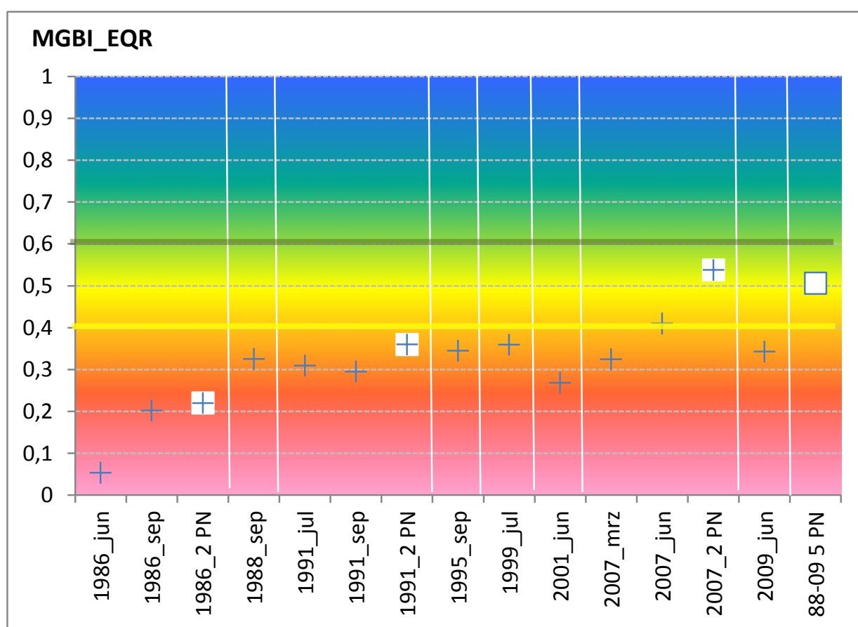
Abb. 48: Zusammenhang EQR_{MGBI\_Subtyp\_Marschen} (vorläufig) und Anzahl der Beprobungen. Datengrundlage NLWKN BOG: Geeste_MS Bramel, Ökologisches Potenzial: Orange = Grenze unbefriedigend/schlecht; gelb = Grenze unbefriedigend/mäßig; grün = Grenze mäßig/gut; blau = Grenze gut/sehr gut. PN 2= Mittelwert aus 2 Probenahmen (saisonal), 5 PN = Mittelwert aus 5 Probenahmen (saisonal & interannuell, Datenreihe 88 – 09). Gelbe Linie vorl. Grenze zu moderat, grüne Linie vorl. Grenze zu gut.
