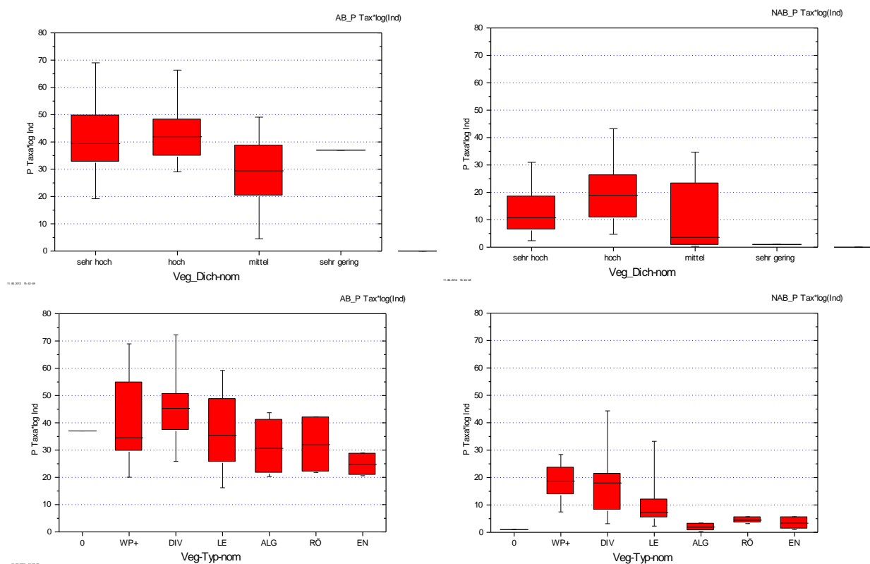
Abb. 31: Richness (Taxazahl * (\log+1 \text{ Ind./Cpue}) ) differenziert nach „Luftatmern“ (Bilder links) und „Nicht-Luftatmern“ (Bilder rechts). Datengrundlage Claus et al. (1994). 0 = keine Unterwasservegetation, WP+ = Wasserpest (und andere), Div = Diverse (Hornkraut, Laichkräuter etc.), Le = höherer Anteil Wasserlinsen, ALG = algendominierte Gewässer, RÖ = höherer Anteil Röhricht, EN = Enteromorpha-Gewässer. Std.Abw. = Standardabweichung.
