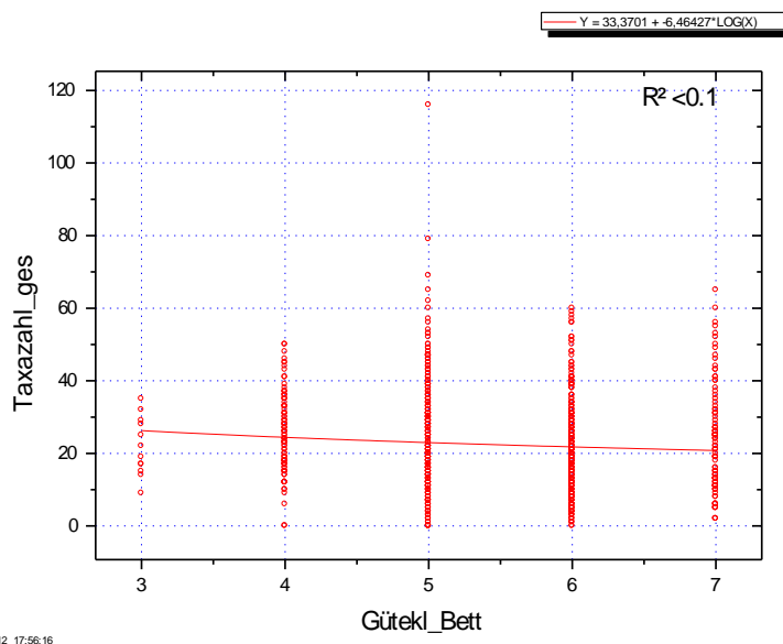
Abb. 23: Zusammenhang von Makrozoobenthostaxazahl (gesamt) und Strukturgüteklassifizierung der Gewässersohle in nicht tideoffenen Marschengewässern in Niedersachsen. Daten NLWKN Stade. Bezeichnung: 7 = vollständig verändert, 6 = sehr stark verändert, 5 = stark verändert, 4 = mäßig verändert, 3 = deutlich verändert, 2 = gering verändert.
