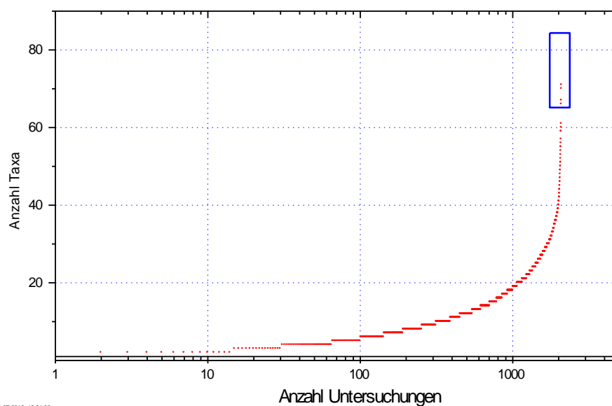
Abb. 44: Spannwerte der Taxazahl/Beprobung in Marschengewässern (Niedersachsen, Bremen, Hamburg, Schleswig-Holstein, N_{\text{ges}} = 2.127 Datenreihen, 1980 – 2011).
