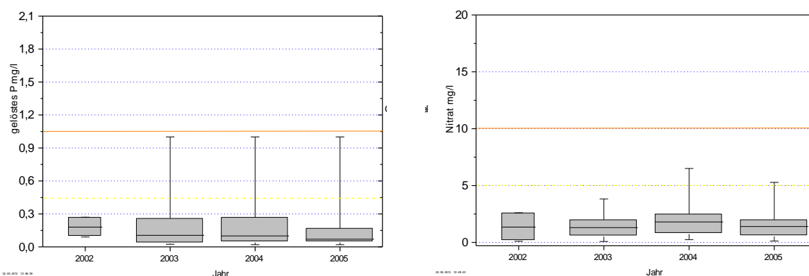
Abb. 8: Räumliche und zeitliche Varianz der Phosphat- und Nitratkonzentration (mg/l) in nicht tideoffenen Marschengewässern im EZG der Tideems und der Wattenmeerküste. Anzahl Messwerte N = 168; Daten NLWKN Aurich. Gelbe Linie: Grenze auffällige Werte, orange Linie: Grenze stark auffällig. Terminologie nach STAWA AURICH 1996.
