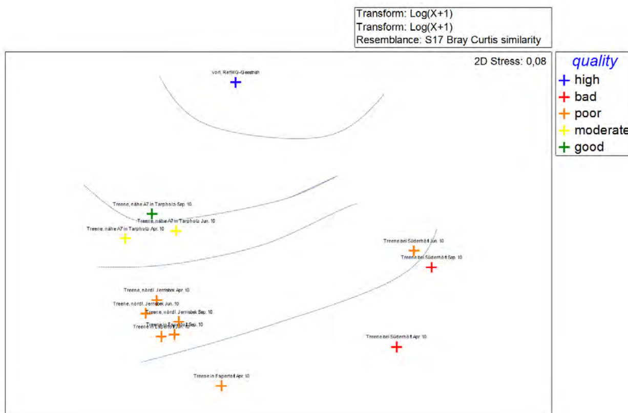
Abb. 49: MDS-Ordinationen auf der Grundlage von Treene sowie Referenzdaten (Arten-Abundanzdaten, Log-transformiert, N = 17 Datenreihen). Gewässer des Subtyps „Geestnah“.
