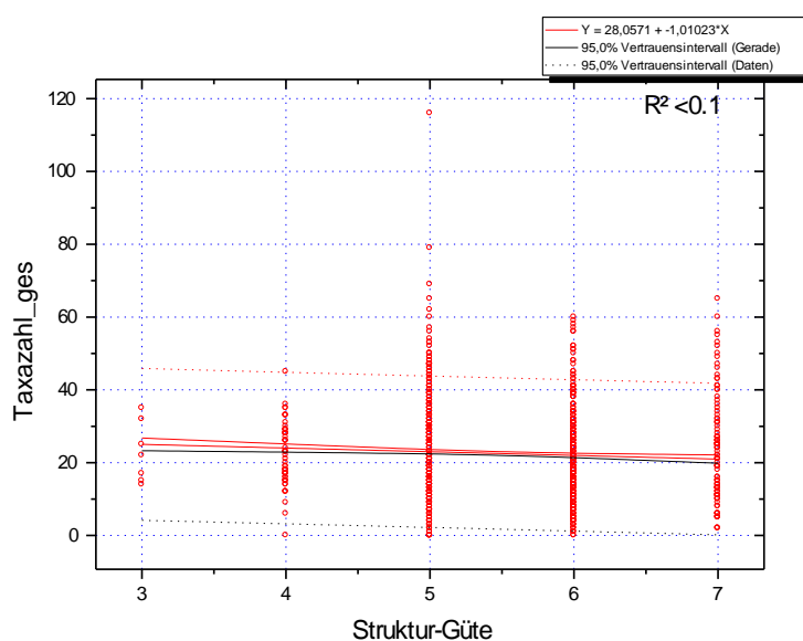
Abb. 22: Zusammenhang von Makrozoobenthostaxazahl (gesamt) und Strukturgüteklassifizierung in nicht tideoffenen Marschengewässern in Niedersachsen. Daten NLWKN Stade. Bezeichnung: 7 = vollständig verändert, 6 = sehr stark verändert, 5 = stark verändert, 4 = mäßig verändert, 3 = deutlich verändert, 2 = gering verändert.
