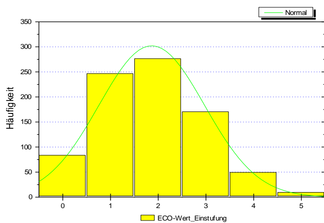
Abb. 40: Häufigkeitsverteilung der Eco-Wert-Kategorien bezogen auf das dokumentierte Gesamtspektrum der Wirbellosentaxa in nicht tideoffenen Marschengewässern (Datenquellen: BOG-NLWKN, SBUVE HB, BSU HH, LLUR SH, Literaturdaten; Zeitraum 1950 – 2011; alle Gruppen, inkl. Diptera, Oligochaeta). Zur Beschreibung der Ecowert-Kat s. Tab. 22.
