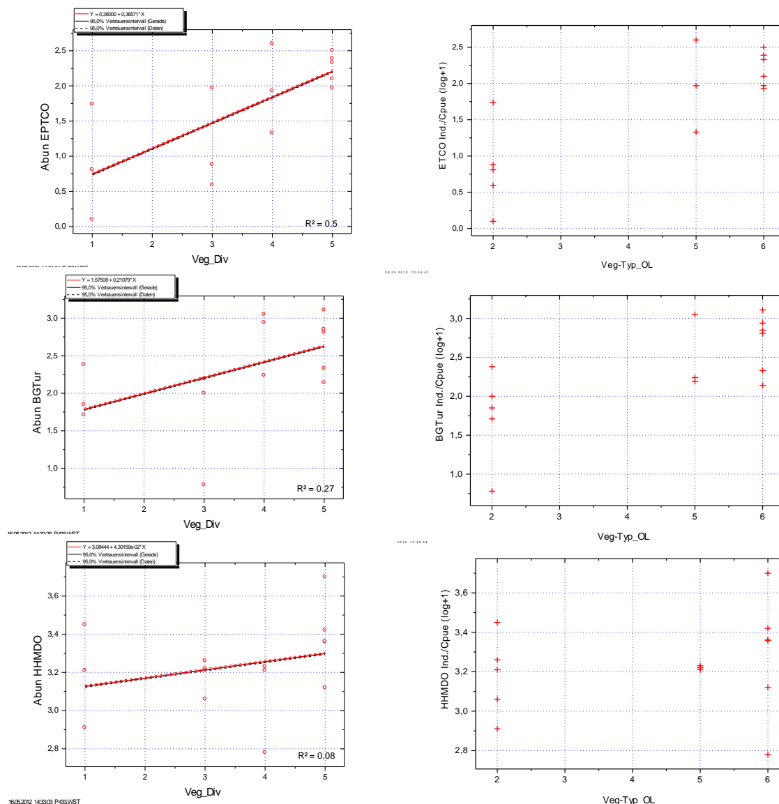
Abb. 27: Darstellung Zusammenhang zwischen Vielfalt und „Typ“ der submersen Vegetation (Veg.-Div., Veg.-Typ) und Makrozoobenthos-Taxazahl auf der Grundlage einer groben Kategorisierung der Makrophytenvariablen. Datenquelle: Gewässer im EZG Küste, Ems, Focke & Kiel (2008). Veg.-Div: 1 = niedrig – 5 sehr hoch. Veg.-Typ. 2 = Röhricht, 5 = Wasserpest dominiert, 6 = verschiedene Arten (Laichkräuter, Hornkraut etc.). ETOC = Ephemeroptera, Trichoptera, Odonata, Coleoptera; BGTur = Bivalvia, Gastropoda, Turbellaria, HHMDO= Hirudinea, Heteroptera, Megaloptera, Diptera, Oligochaeta, auf die Darstellung der Crustacea wurde hier verzichtet.
