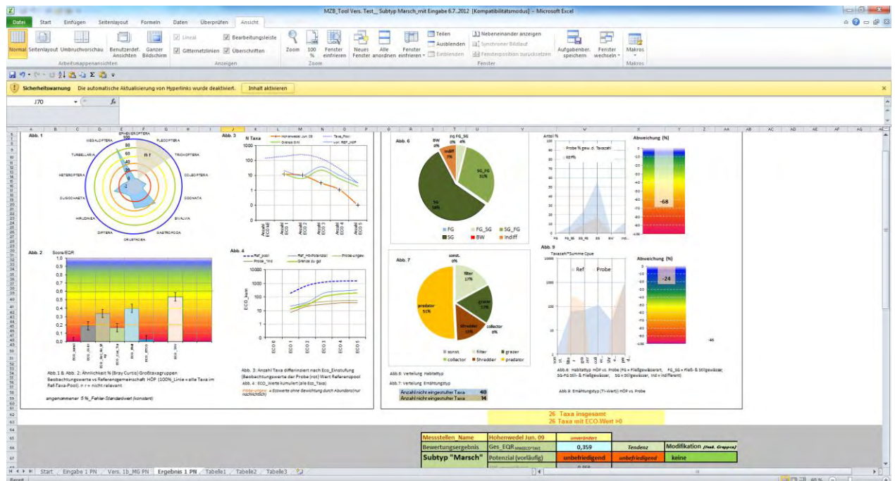
Abb. 53: Ergebnisblatt Subtyp „Marschen“
