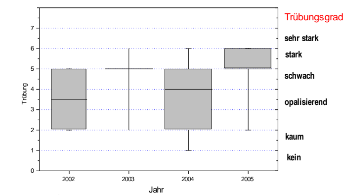
Abb. 6: Räumliche und zeitliche Varianz des Trübungsgrads in tidegeschossenen Marschengewässern im EZG der Tideems und der Wattenmeerküste. Anzahl Messwerte N = 168; Daten NLWKN Aurich
