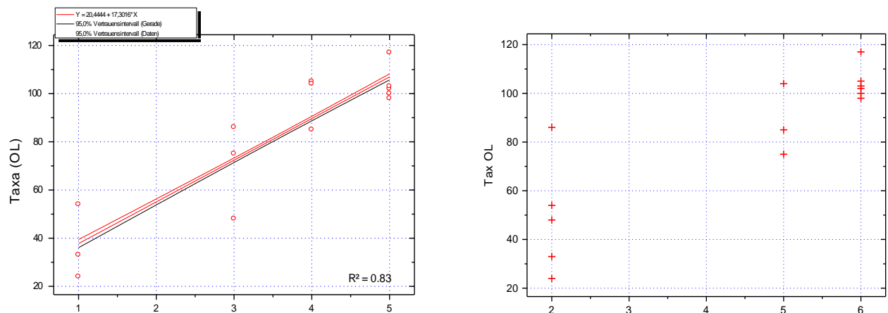
Abb. 26: Darstellung Zusammenhang zwischen Vielfalt und „Typ“ der submersen Vegetation (Veg.-Div., Veg.-Typ) und Makrozoobenthos-Taxazahl auf der Grundlage einer groben Kategorisierung der Makrophytenvariablen. Datenquelle: Gewässer im EZG Küste, Ems, Focke & Kiel (2008). Veg.-Div: 1 = niedrig – 5 sehr hoch. Veg.-Typ. 2 = Röhricht, 5 = Wasserpest dominiert, 6 = verschiedene Arten (Laichkräuter, Hornkraut etc.)
