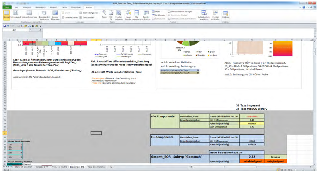
Abb. 54: Ergebnisblatt Subtyp „Geestnah“
